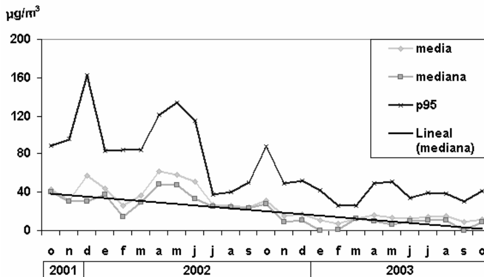
Figura 6: Comportamiento de índice de acidez. Estación de Monitoreo Centro Habana. Octubre 2001 - Octubre 2003.
