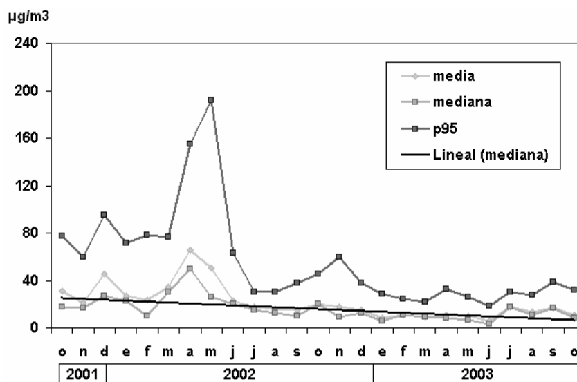
Figura 4: Comportamiento del dióxido de azufre. Estación de monitoreo. Centro Habana. Octubre 2001 – Octubre 2003.
