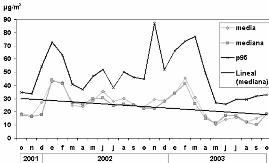
Figura 5: Comportamiento del dióxido de nitrógeno. Estación de monitoreo. Centro Habana. Octubre 2001 - Octubre 2003.
