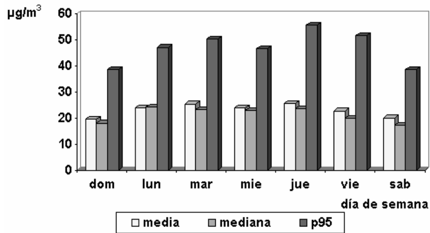
Figura 3: Concentraciones de dióxido de nitrógeno por días de la semana. Centro Habana. Octubre 2001 - Octubre 2003.
