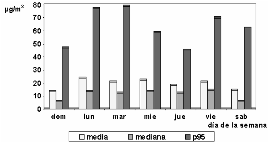
Figura 2: Concentraciones de dióxido de azufre por días de la semana. Centro Habana. Octubre 2001 - Octubre 2003.
