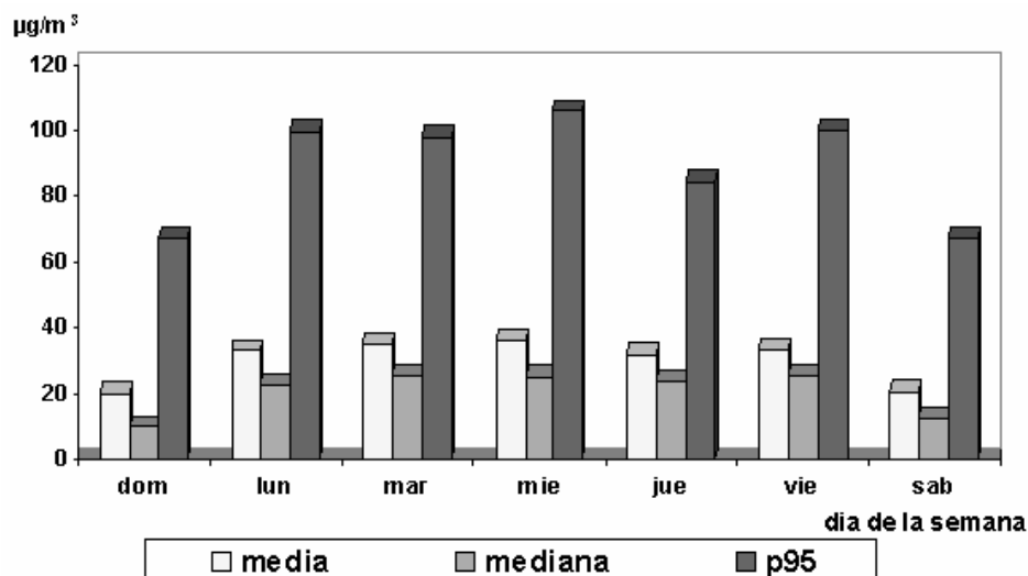
Figura 1: Comportamiento de índice de acidez por días de la semana. Estación de Monitoreo Centro Habana. Octubre 2001 – Octubre 2003.
