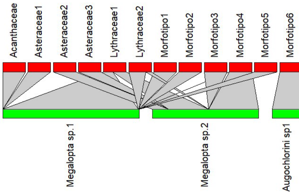
Figura 2. Red bipartida que expone la interacción insecto-planta de Megalopta sp.1 , Megalopta sp.2 y Augochlorini sp.1 . Se presenta en dos ejes ordenados en función del número decreciente de interacciones. El eje verde corresponde a las abejas y su longitud representa la abundancia de cada especie al momento del muestreo, de acuerdo a sus capturas en la trampa de luz.
